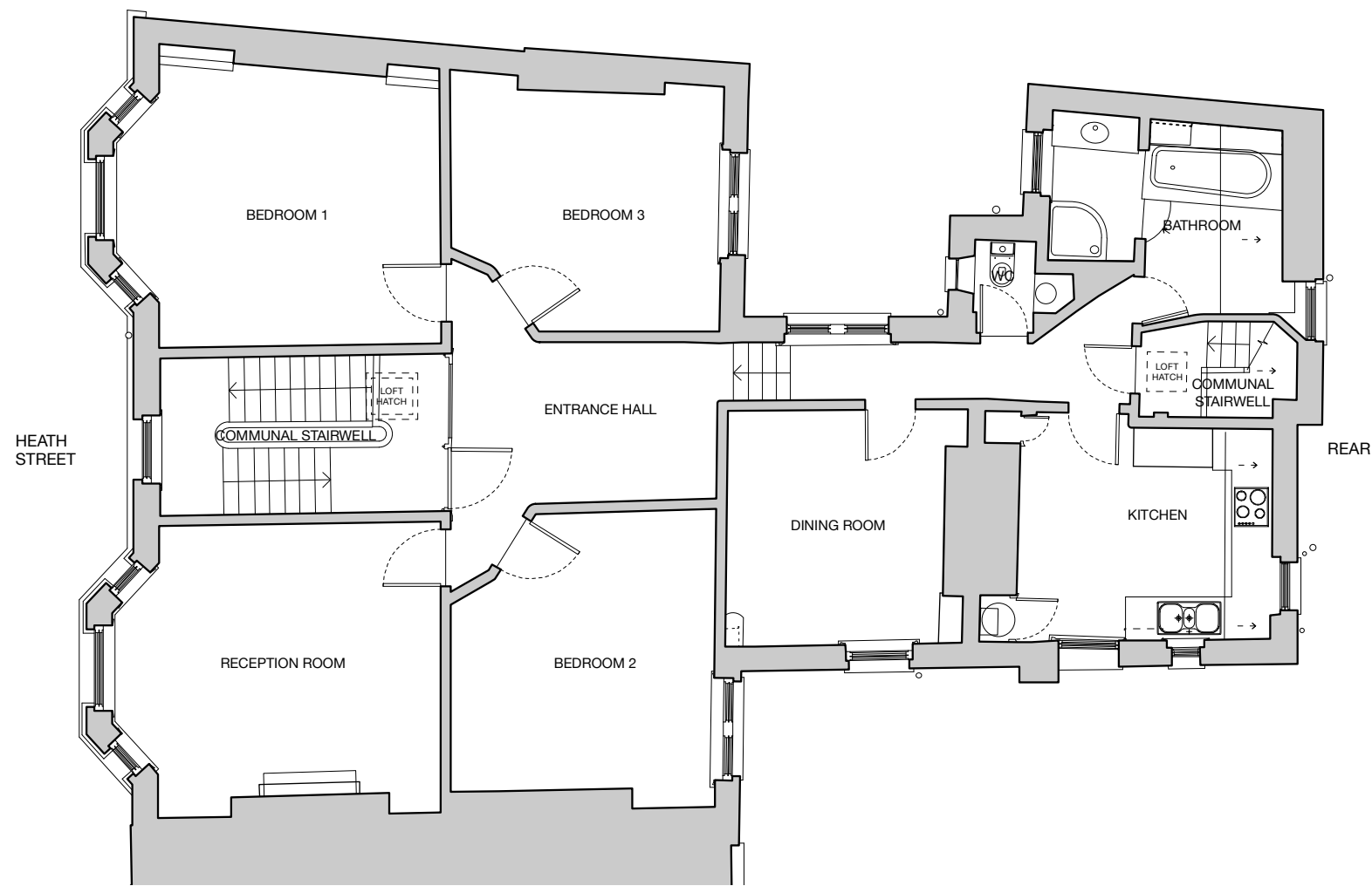
FP Floor Plan Existing Scale: 1:100
