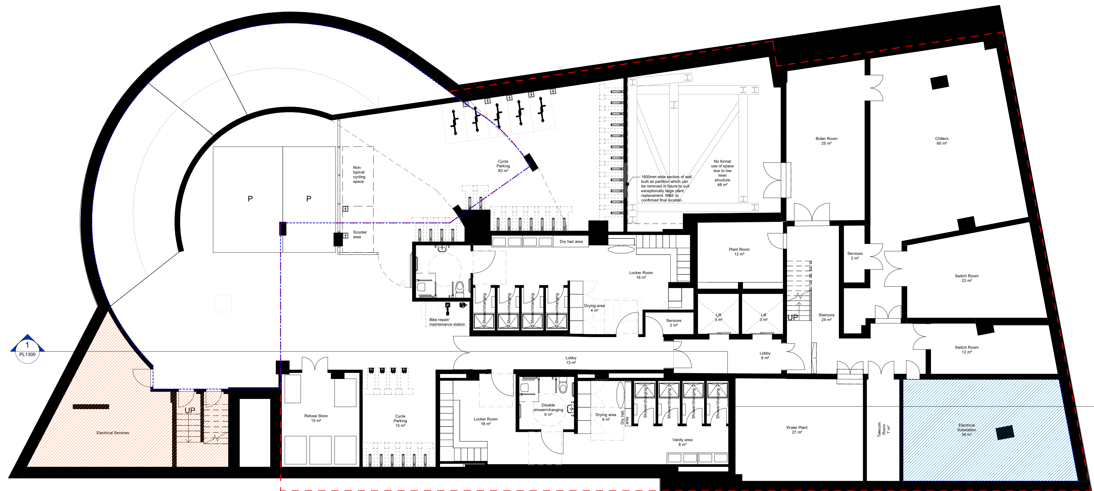
1 -01 - Basement 1 : 100
