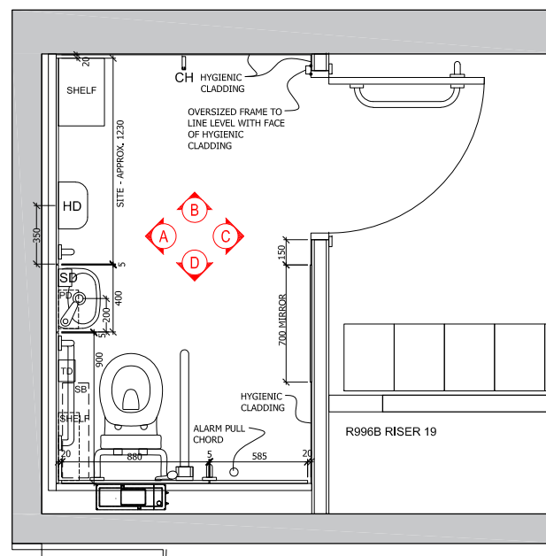
1 ACCESSIBLE WC PLAN 1:20
