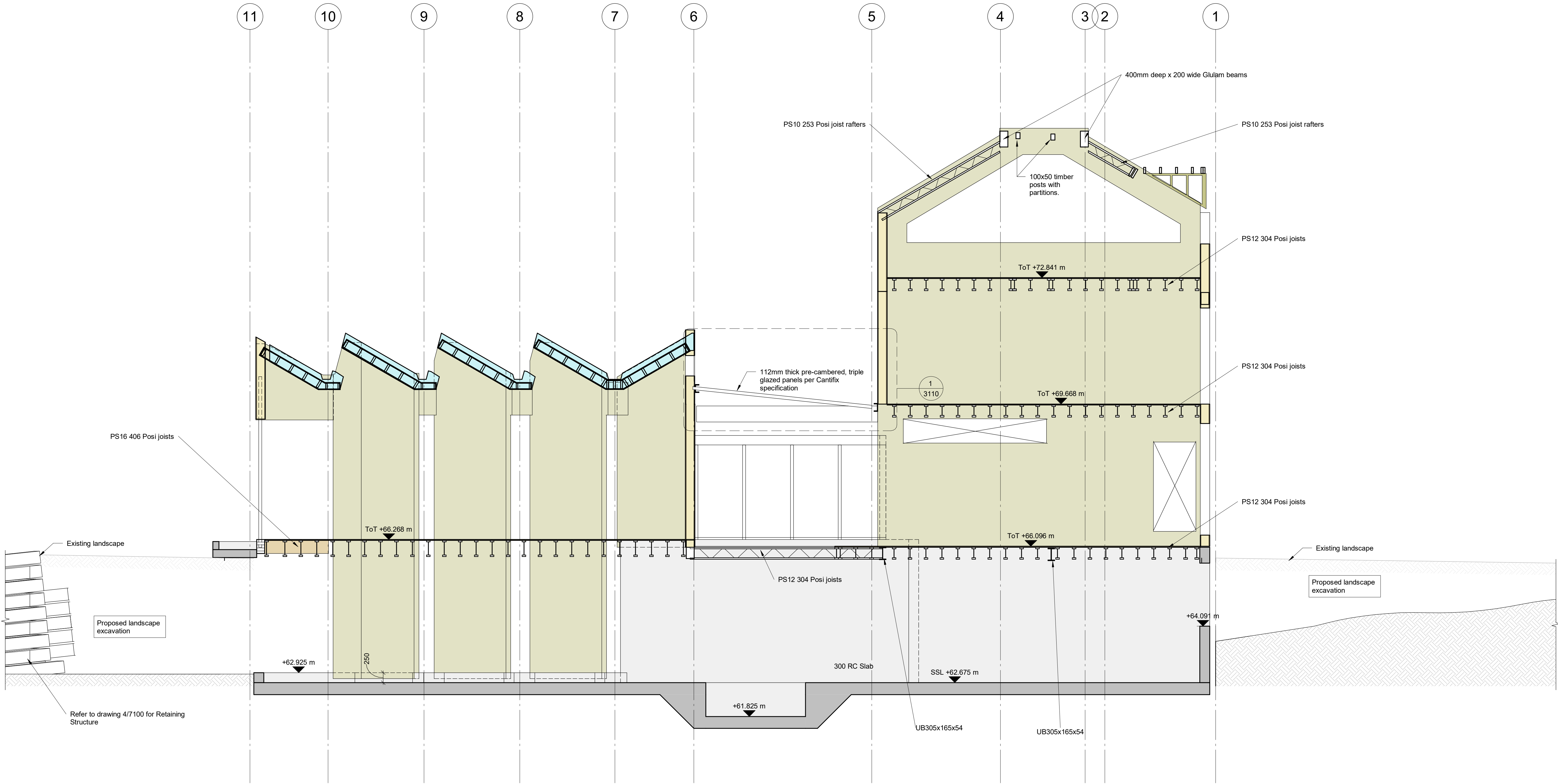
SECTION B-B SCALE: 1 : 50
