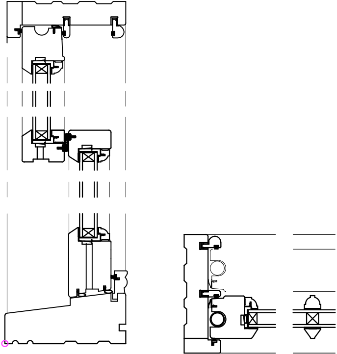
HEAD & CILL 1:5 JAMB 1:5
