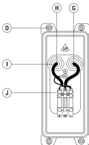
Durchverdrahtung Through wiring
