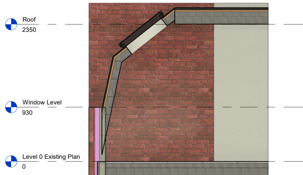
3 Section 4 - Callout 1 1 : 25
