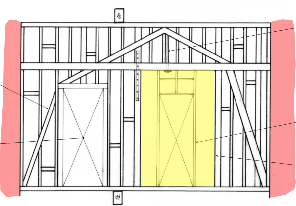
Elevation A-A
