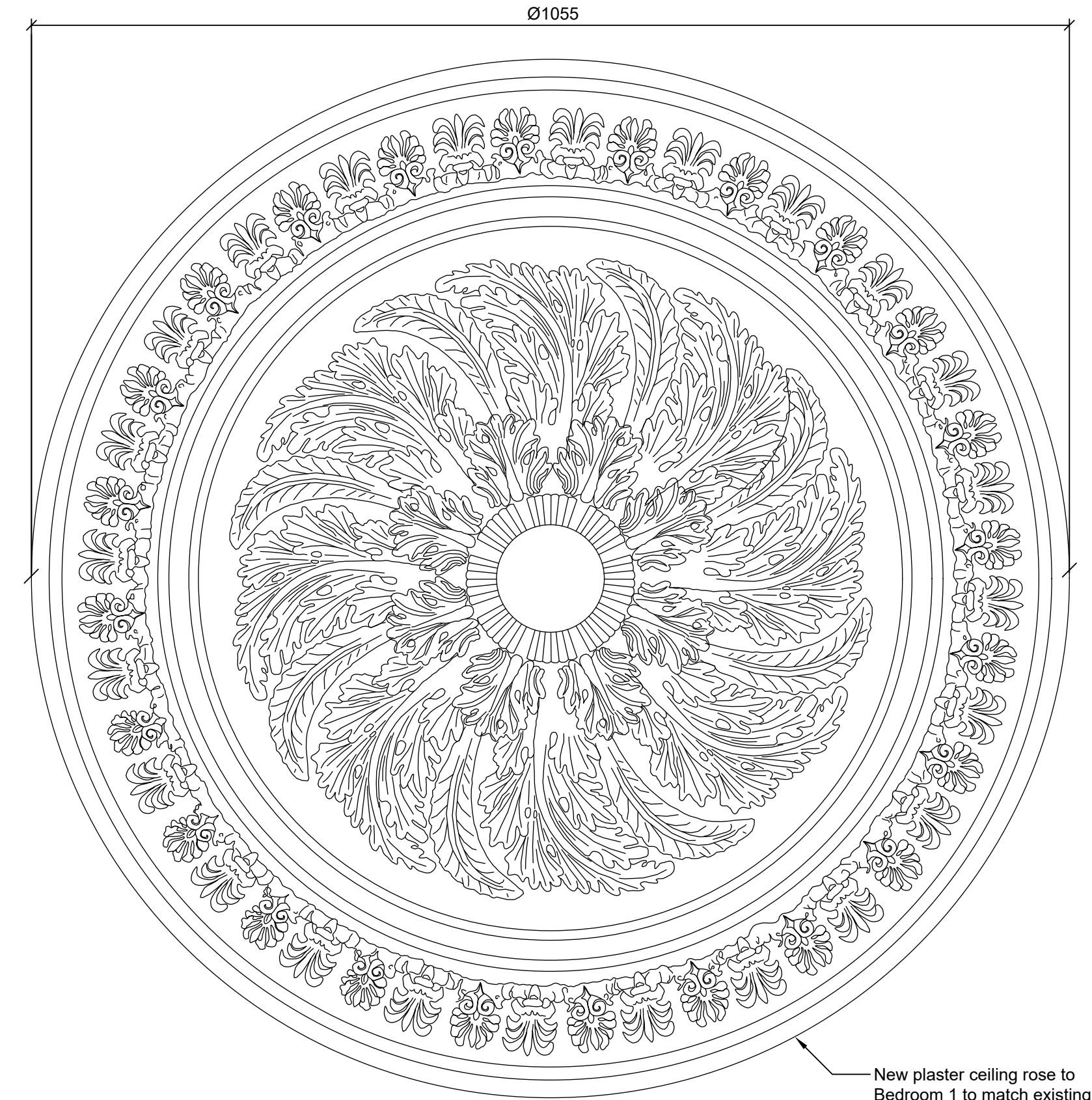
01 Ceiling Rose 3005 1:5 @ A3
