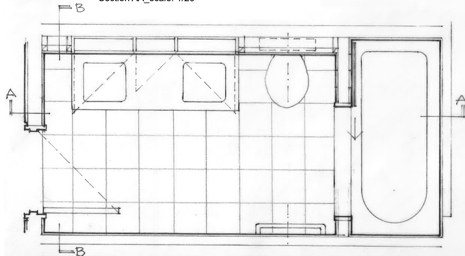
Plan_scale: 1/20
