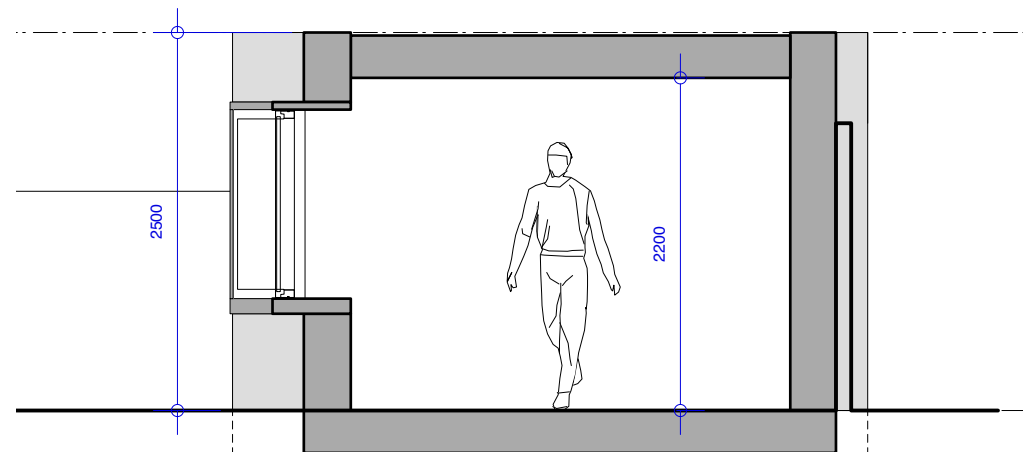
3 Section AA Scale: 1:50
