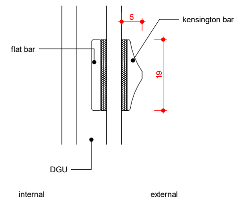
6 Detail 4 1 : 1
