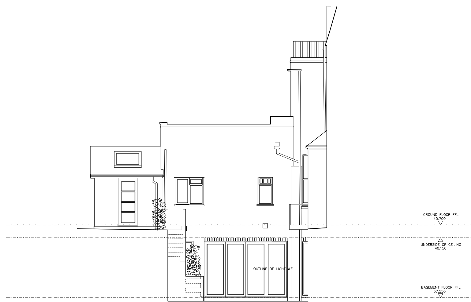
003 SIDE ELEVATION
