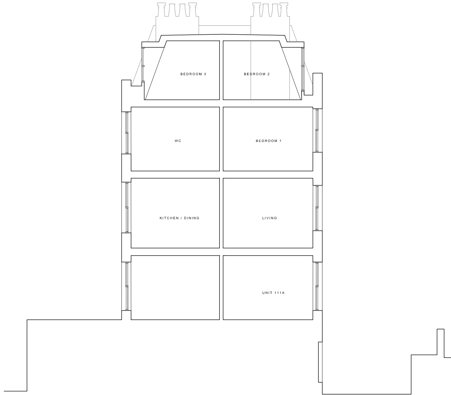
1 Existing Section A-A 1:100
