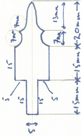
GLAZING BAR
