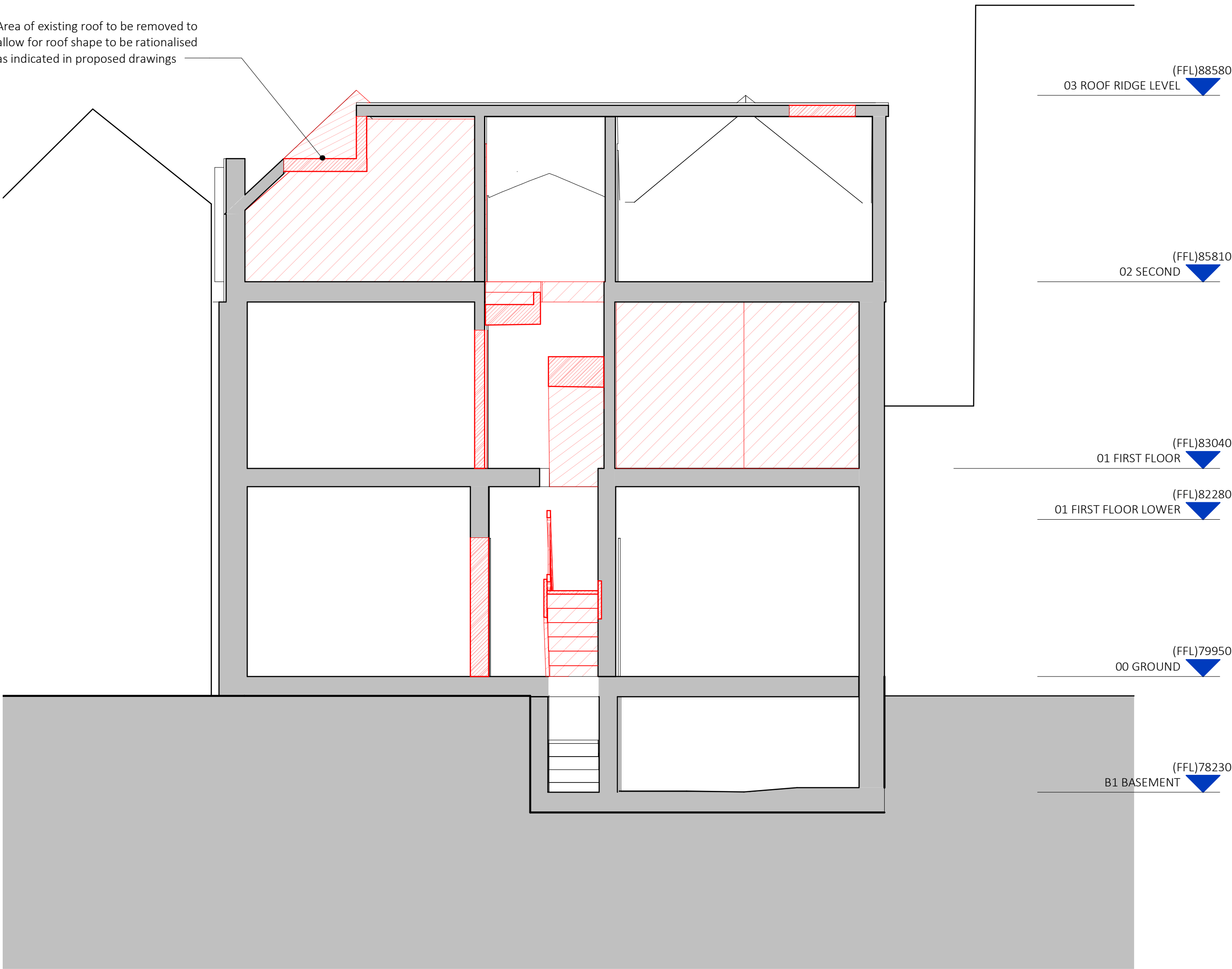
1 1 : 50 EXISTING SECTION B-B
