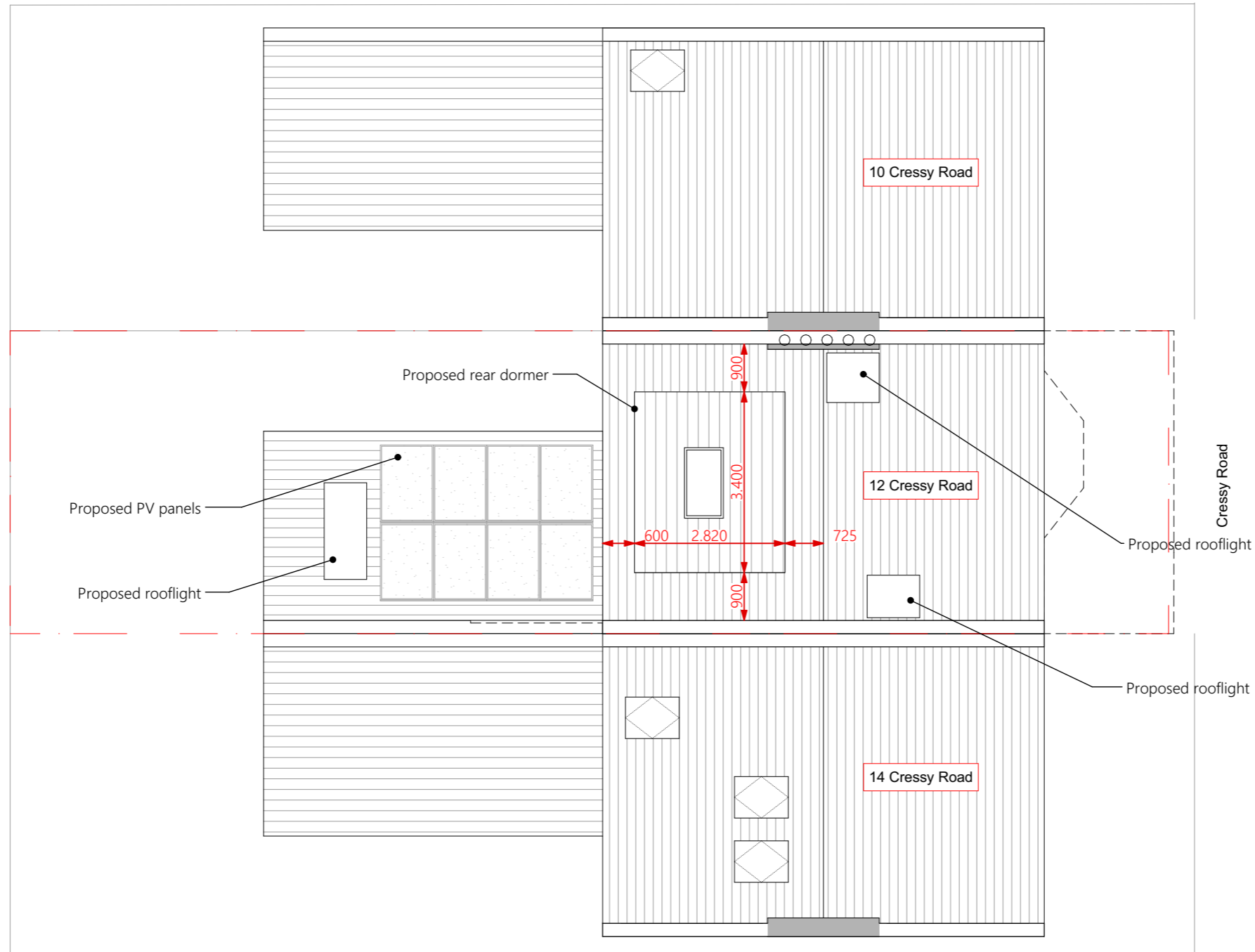
Site Plan 1:100
