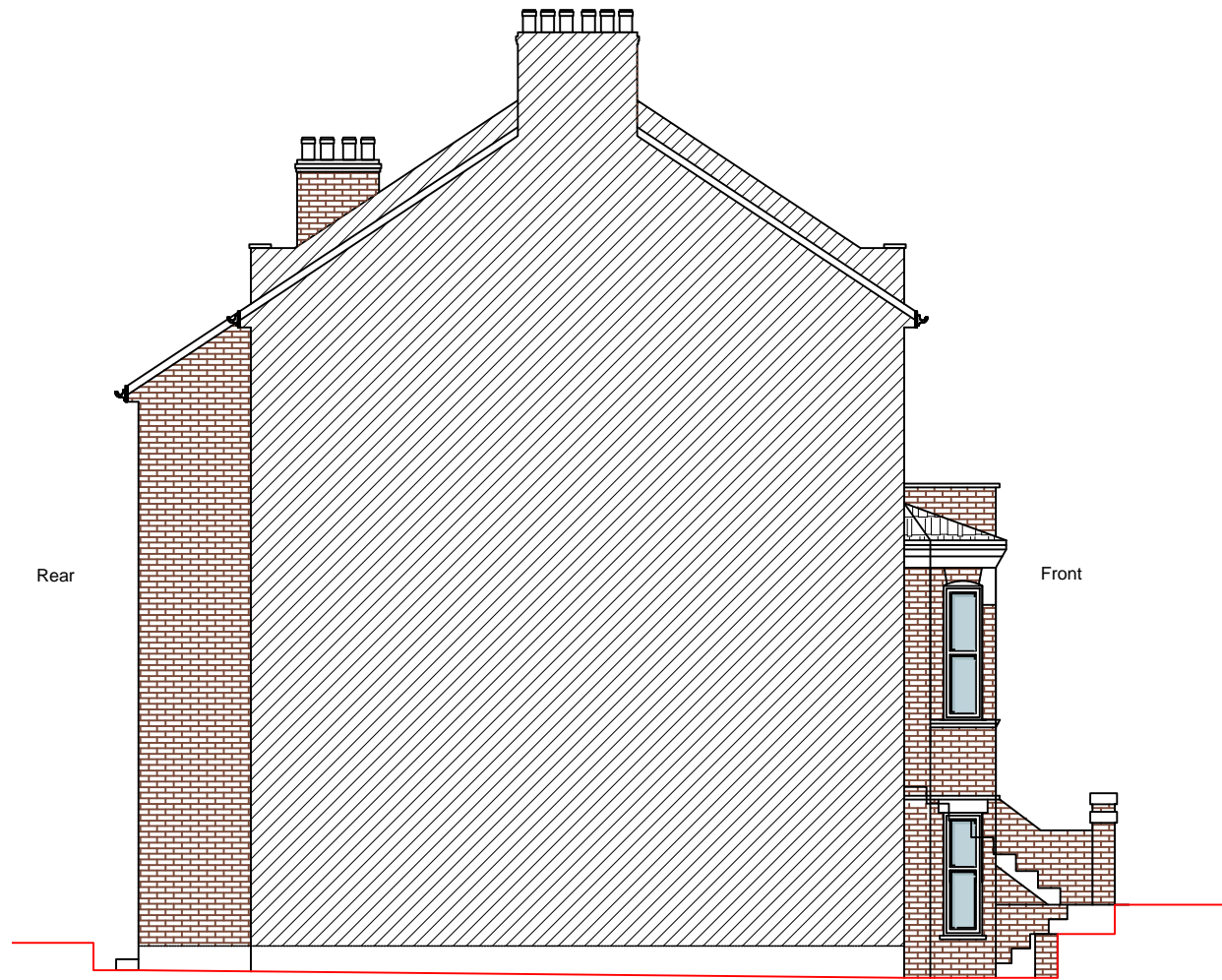
EXISTING FLANK ELEVATION
