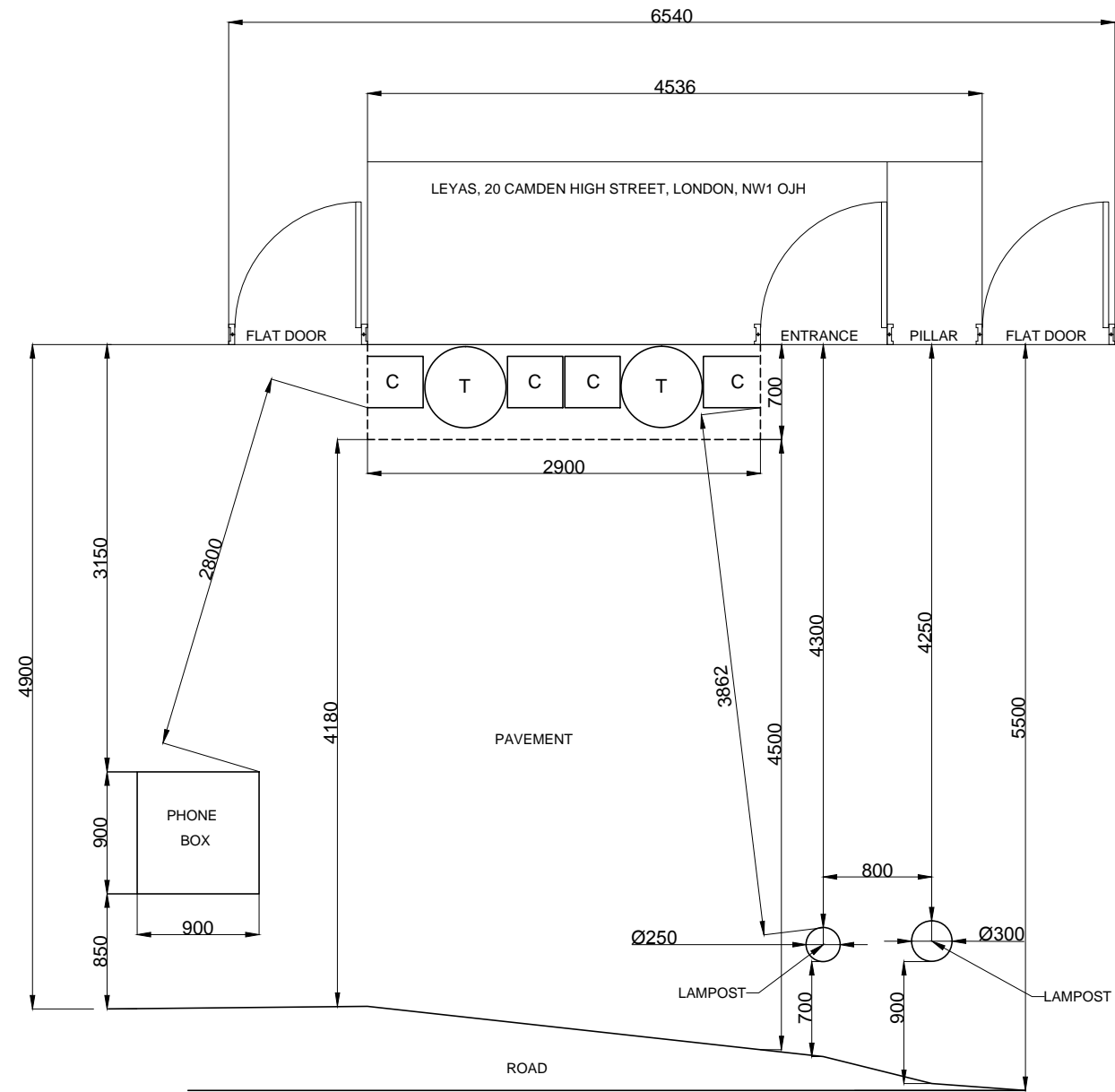
PLAN 1:50
