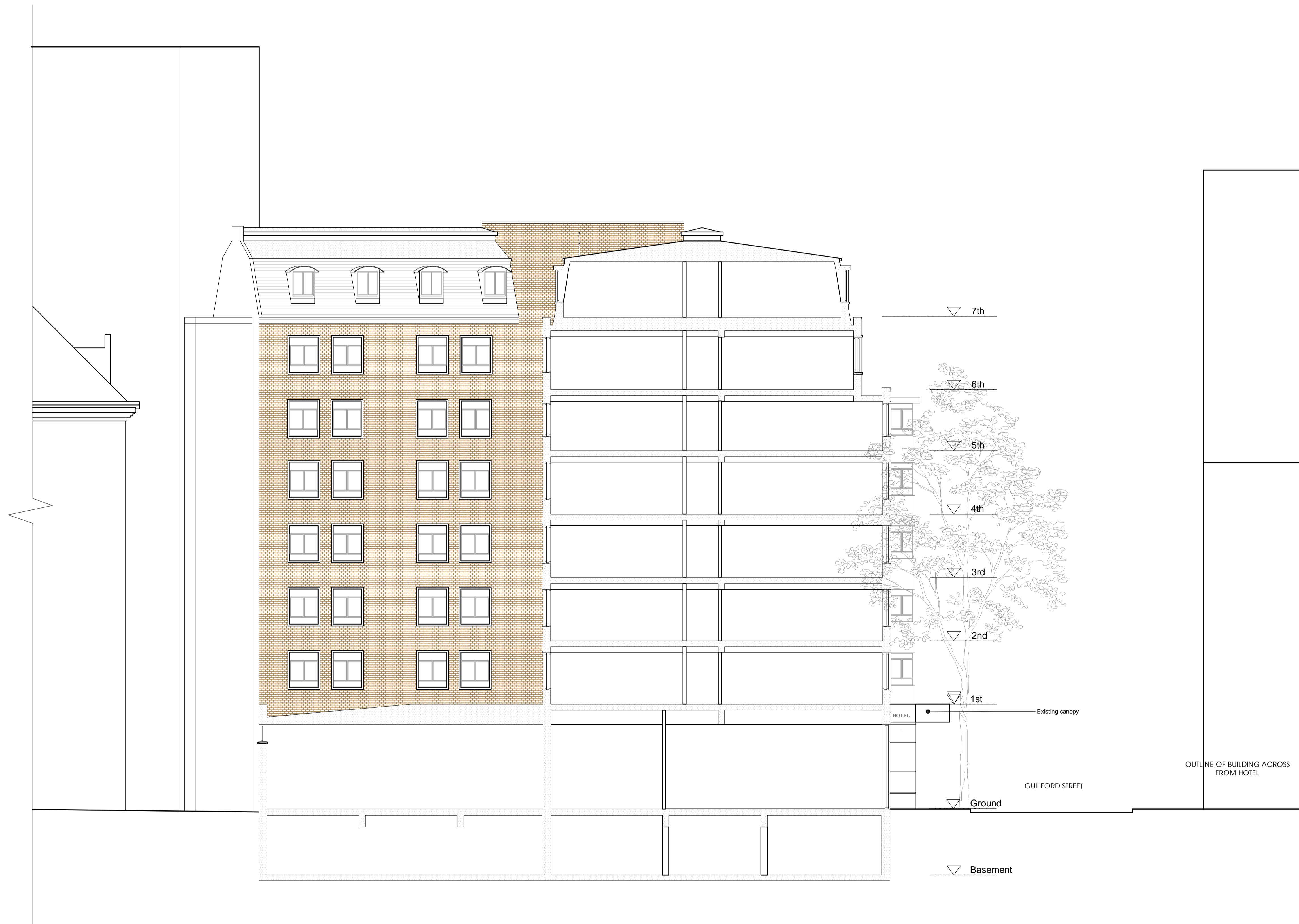
1 SECTION A-A
