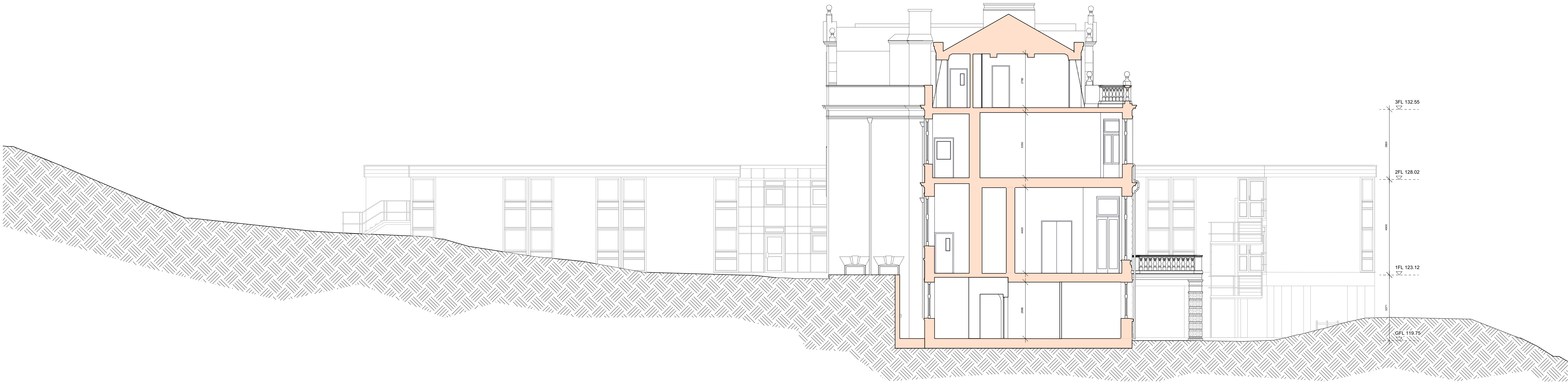
1 EXISTING SECTION F-F PL-09 Scale: 1:100
