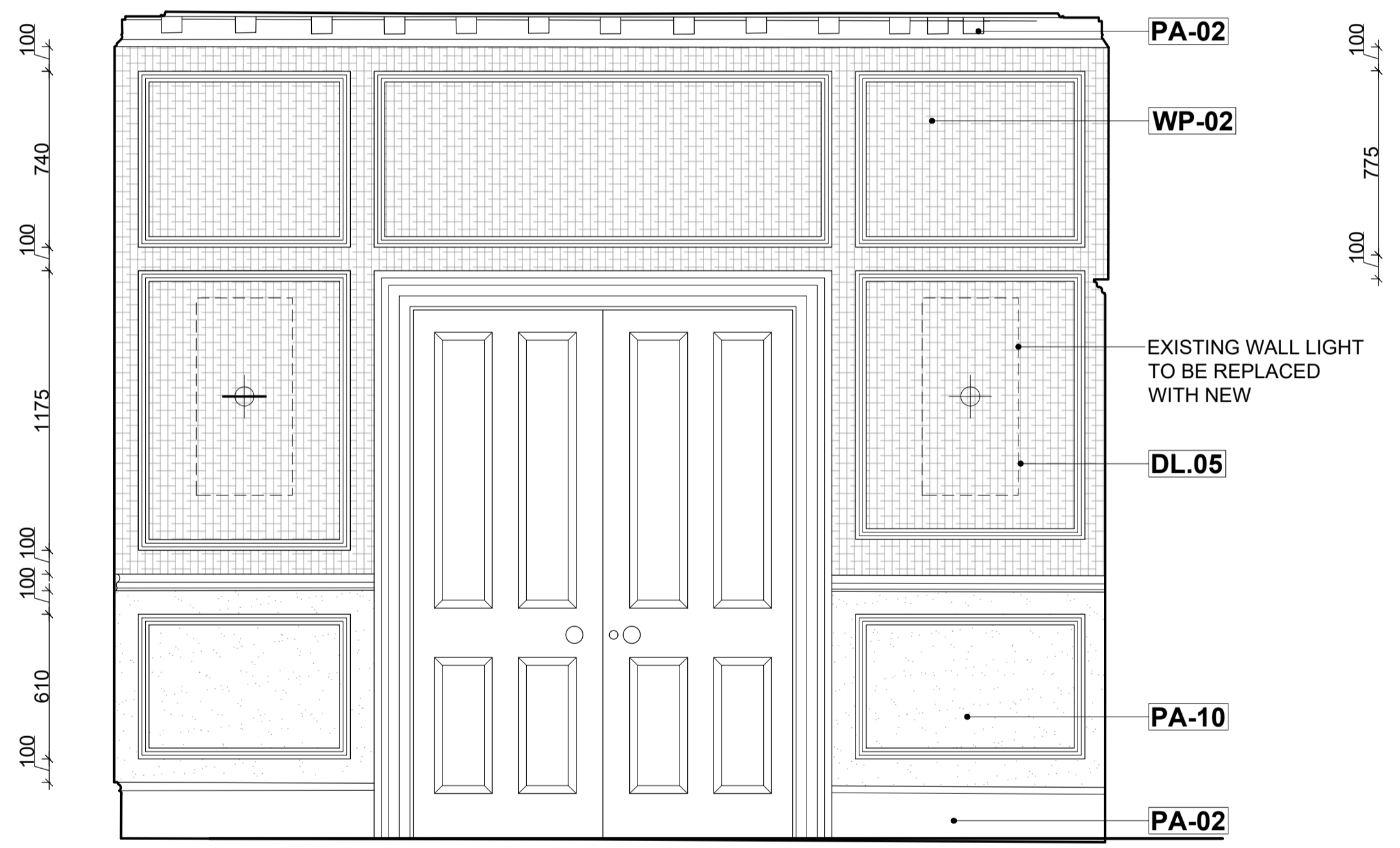
02 ELEVATION G 1:20 @ A1
