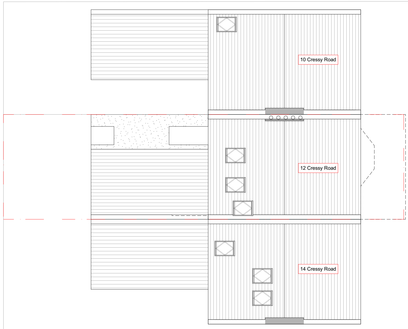
Site Plan ..... 1:100
