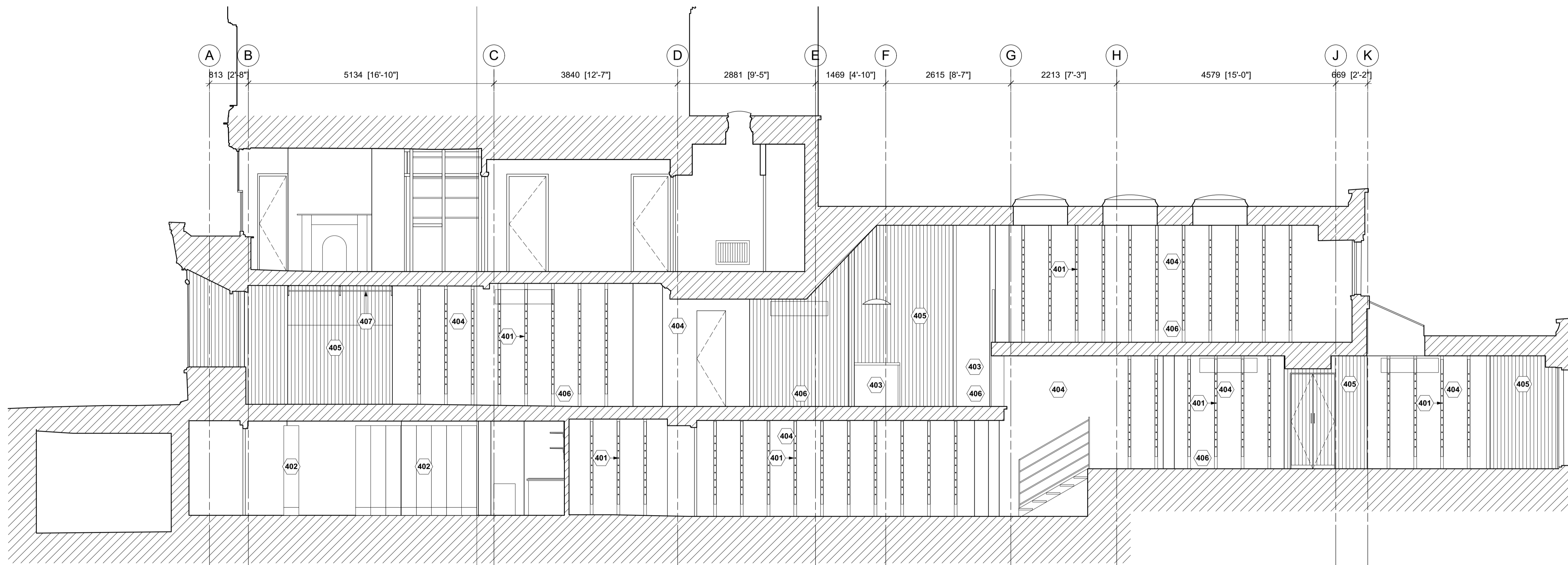
1 SECTION 02 PL401 SCALE: @A1 1:50
