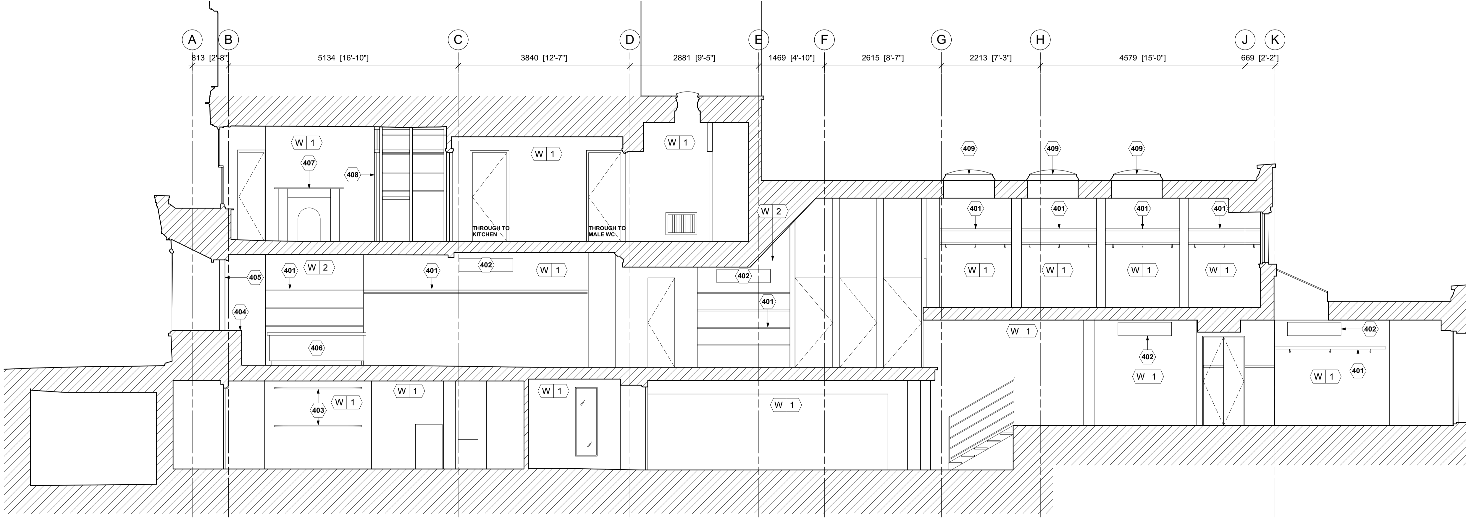
1 EXISTING SECTION 02 EX401 SCALE: @A1 1:50
