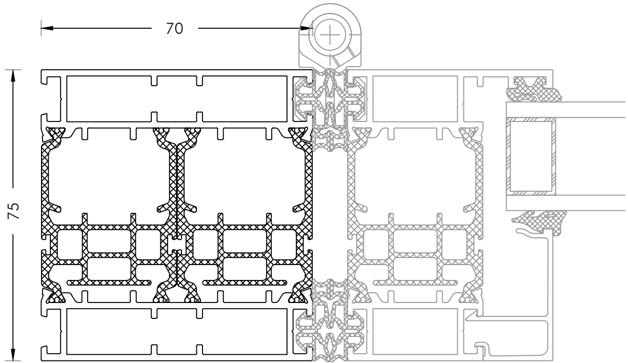
70mm Jamb
