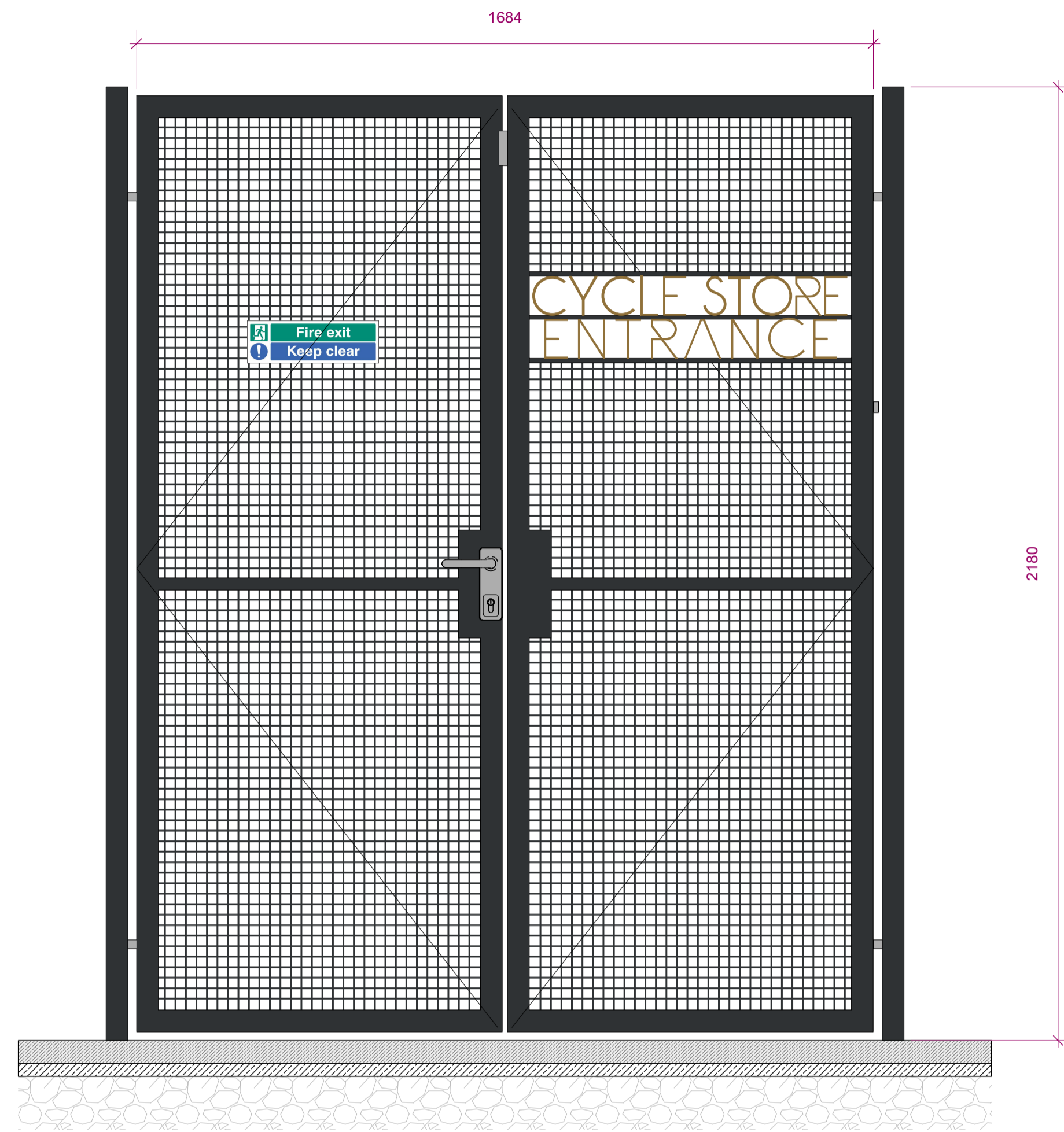
01 CYCLESTORE ENTRANCE DOOR Scale: 1:10
