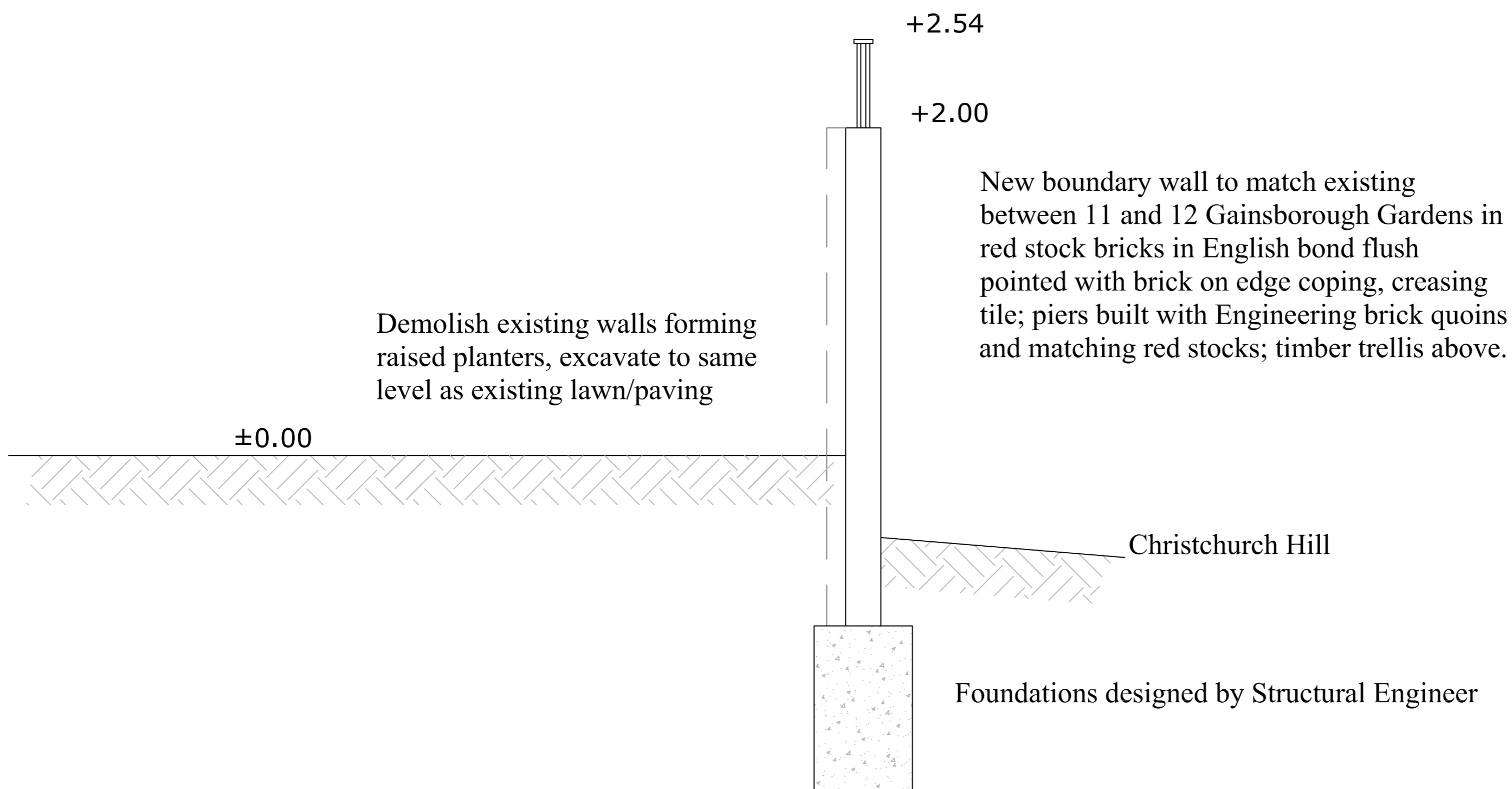
SECTION D-D
