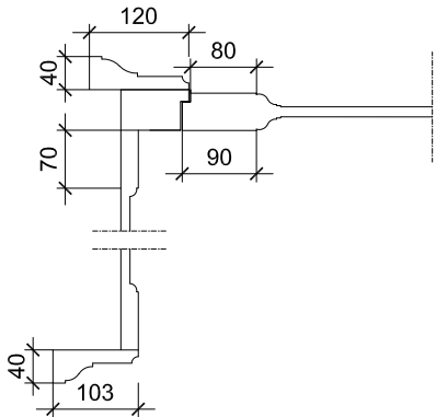
Room G06 - WD03 - Door DG04 + Frame - Wood - SCALE 1:5
