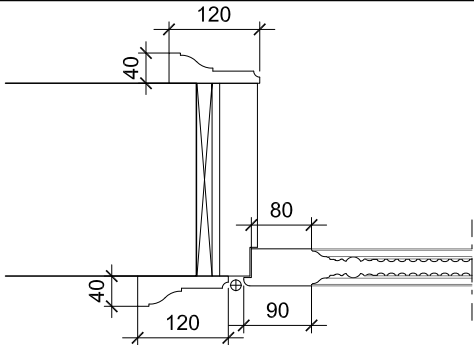
Room G02 - WD03 - Door DG03+ Frame- Wood - SCALE 1:5
