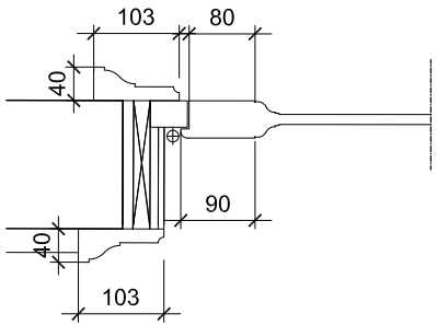
Room G10 - WD03 - Door DG07 + Frame - Wood - SCALE 1:5
