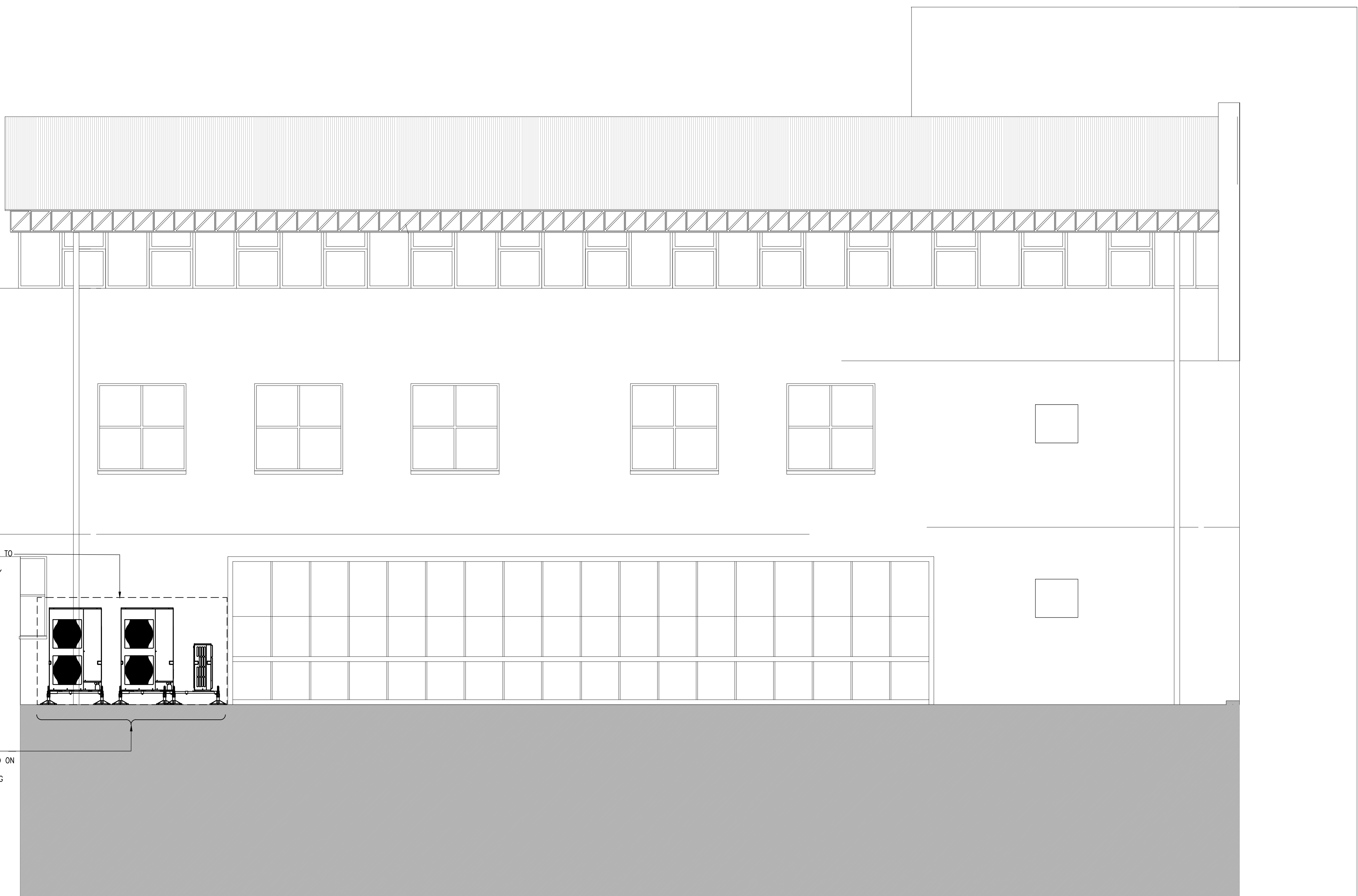
4 Elevation C-C Scale: 1:50
