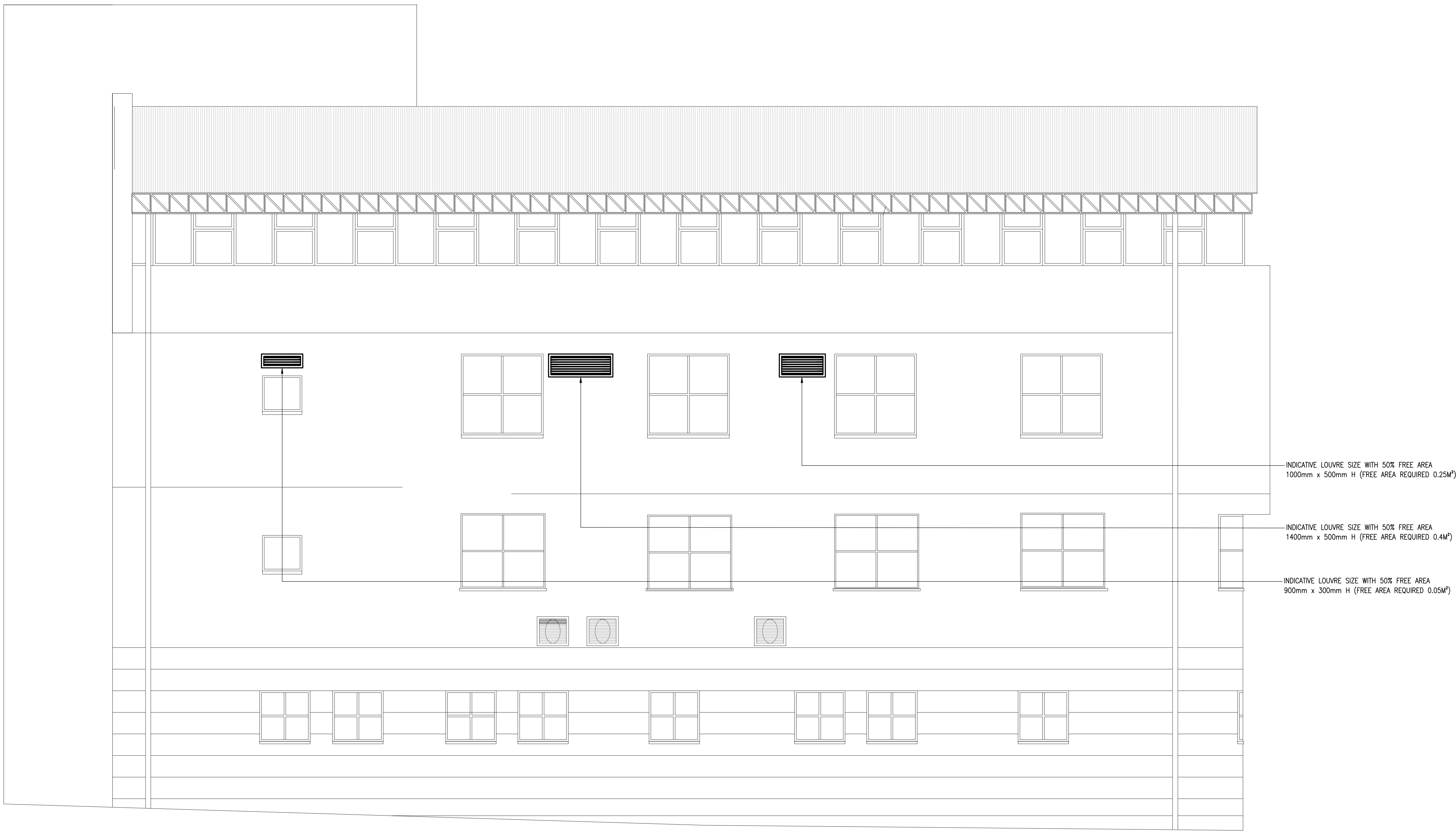
3 Elevation B-B Scale: 1:50
