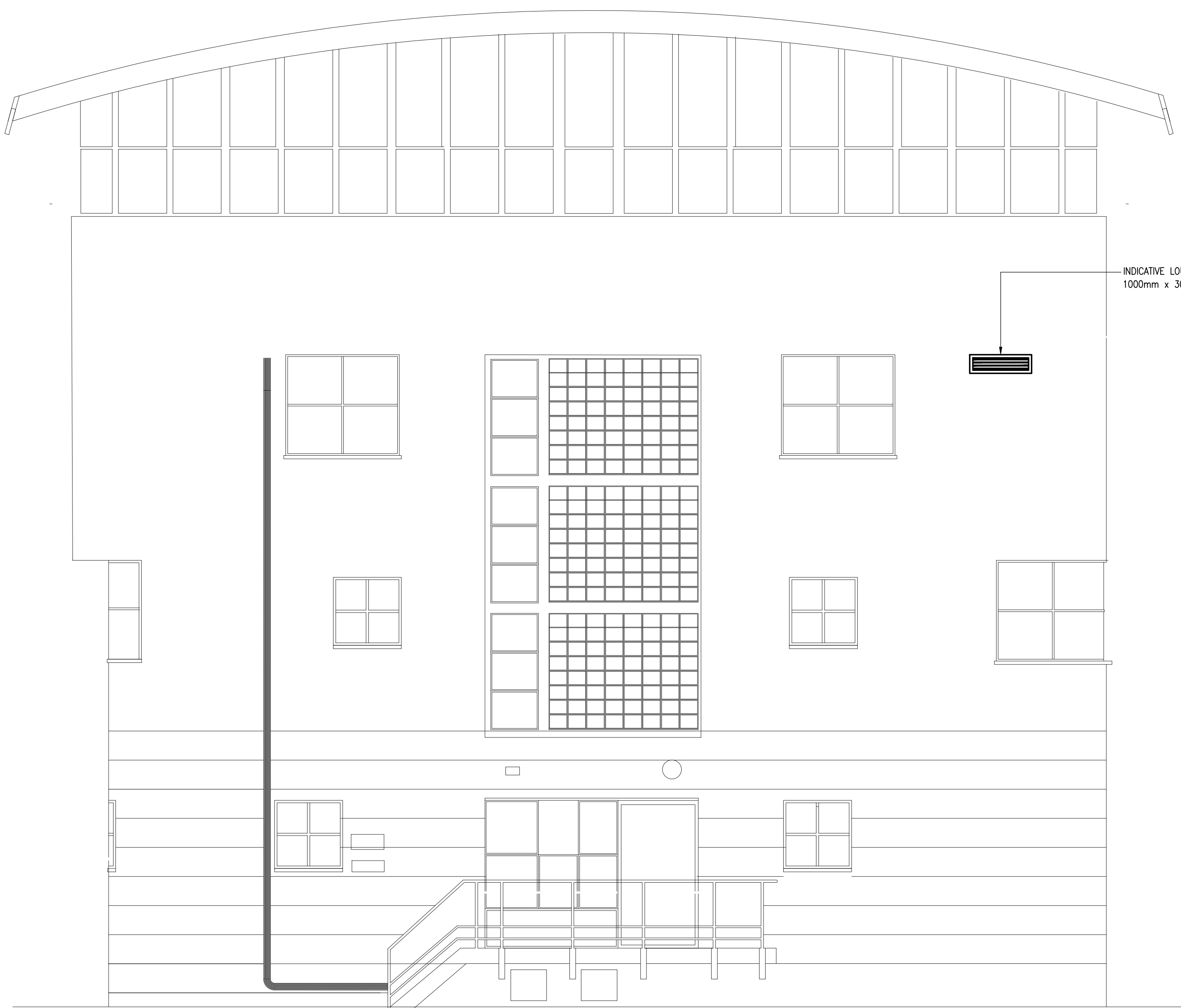
② Elevation A-A Scale: 1:50
