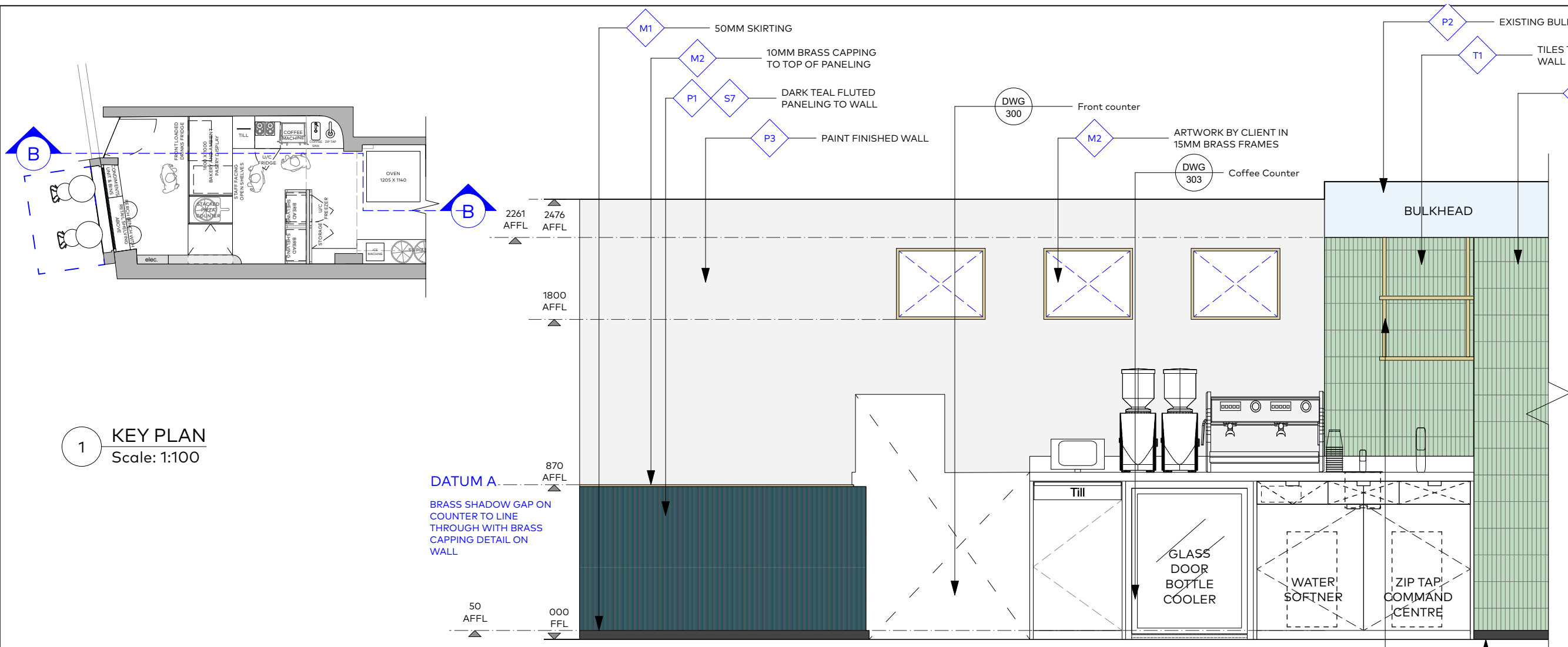
3 SECTION BB Scale: 1:25
