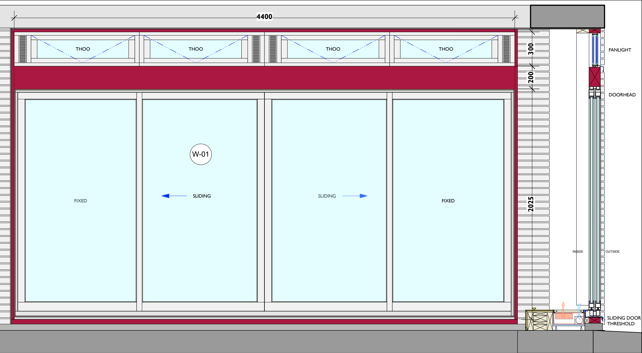
SLIDING DOOR ELEVATION W-01
