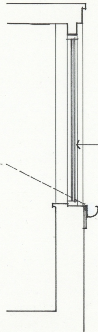
SECTION A-A. SCALE: 1:20 @ A3.
