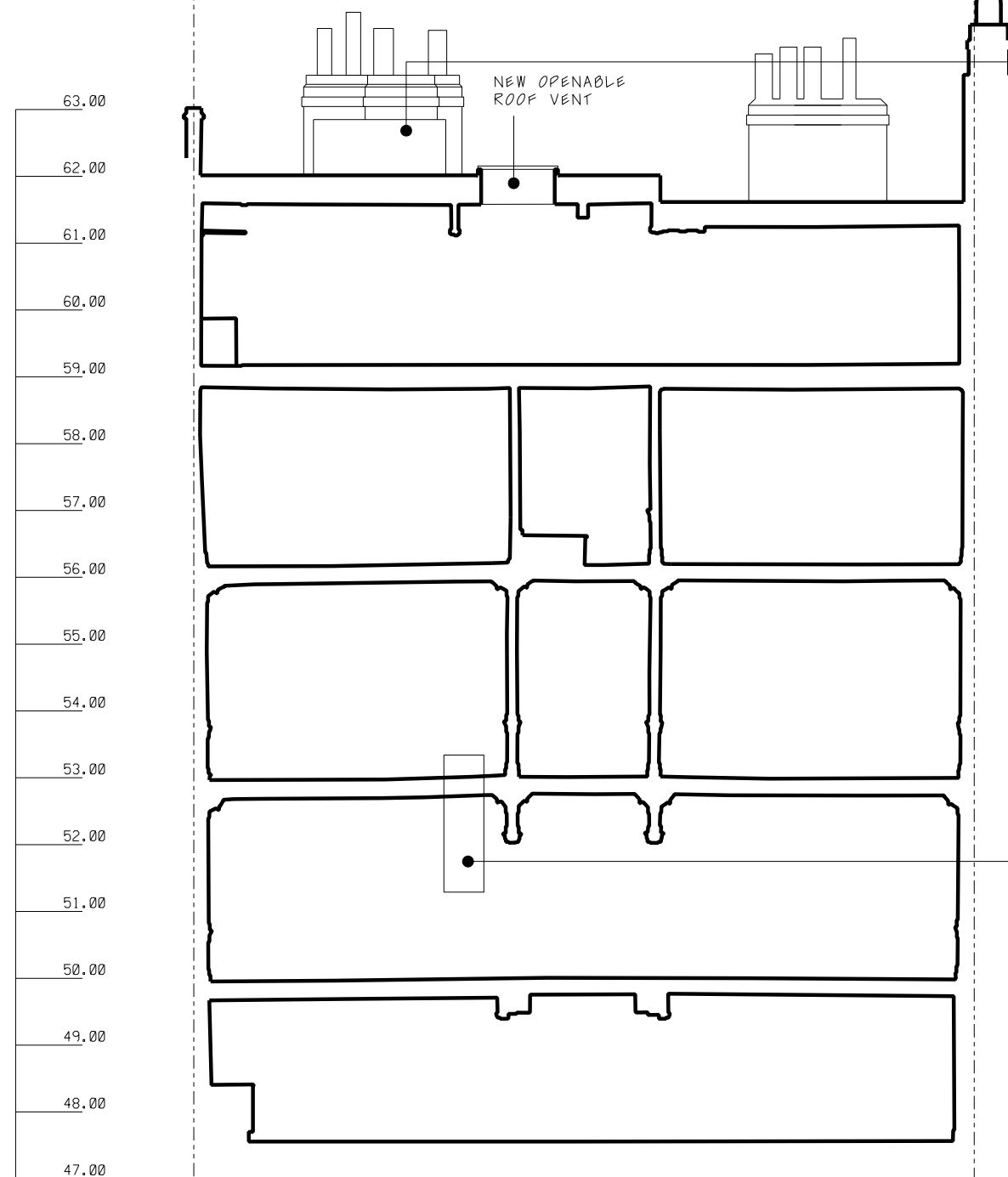
Section A-A
