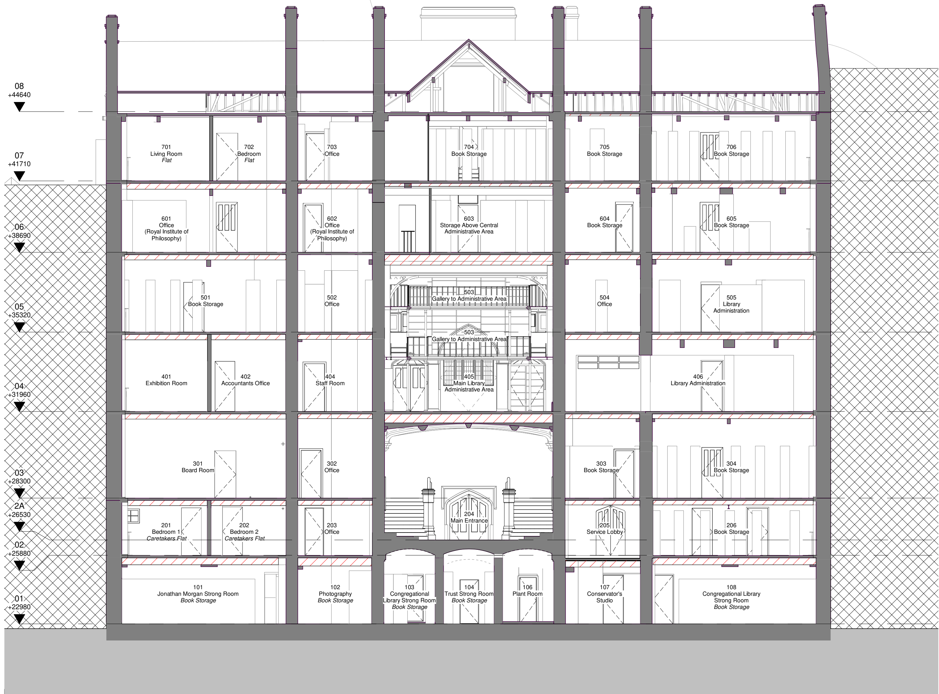
Existing - Section 4 1 : 100
