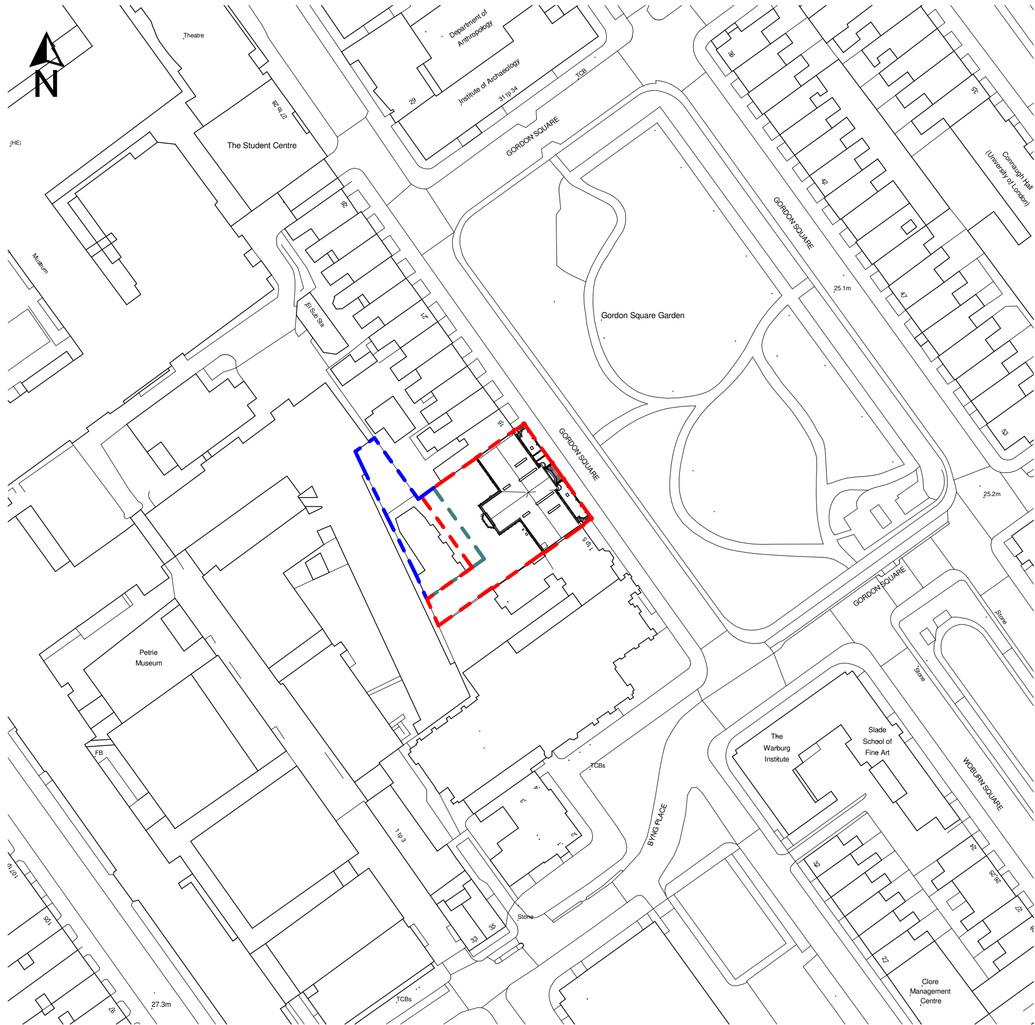
SiteLocationPlan 1 : 1000
