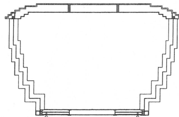
LONGITUDINAL SECTION 1:25
