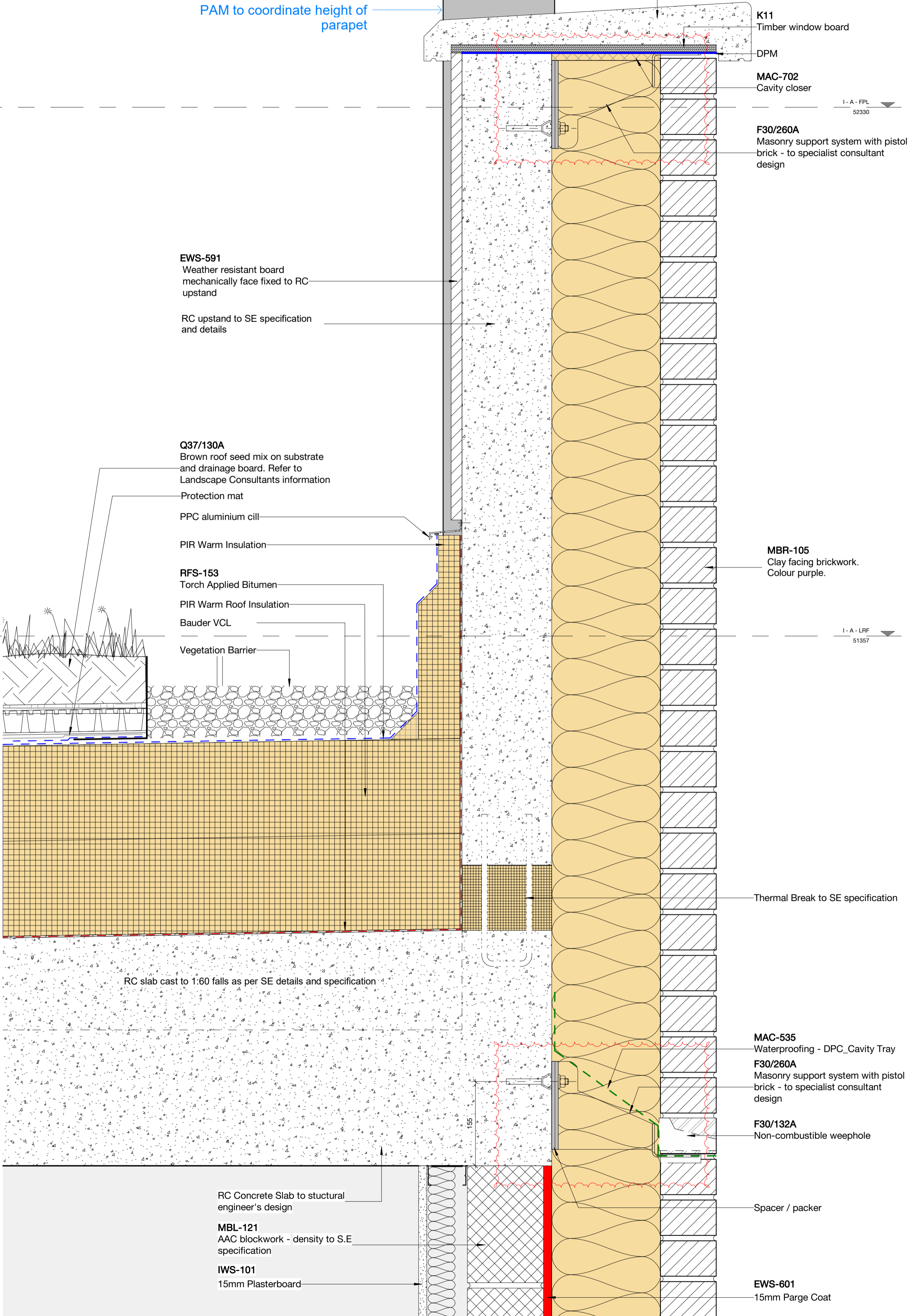
2 LRF Parapet - High Point 1 : 5
