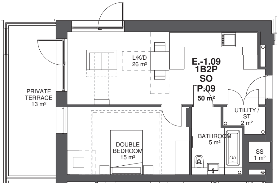
Type P.09 - 1B2P SO
