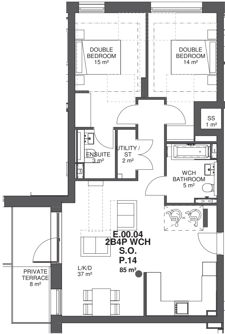
Type P.14 - 2B4P SO
