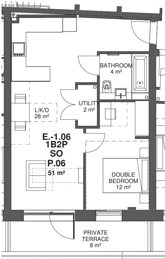
Type P.06 - 1B2P SO
