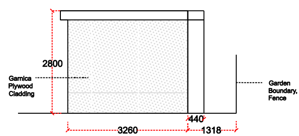
Elevation b-b
