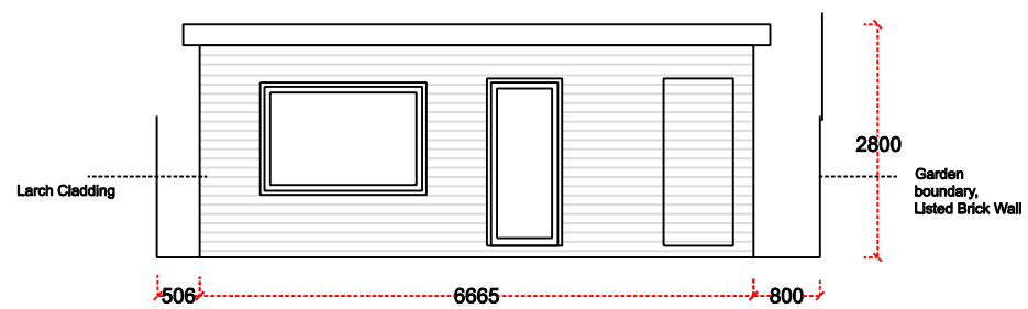
Elevation a-a
