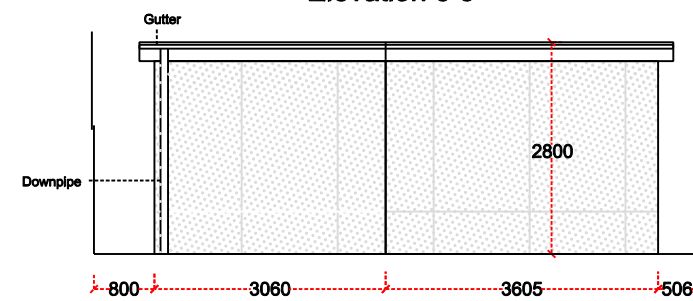
Elevation c-c
