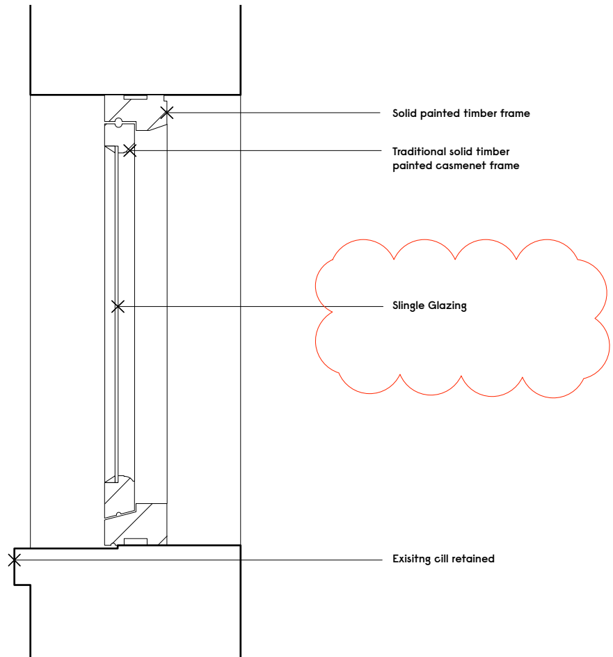
1 Section 1:10 @ A3
