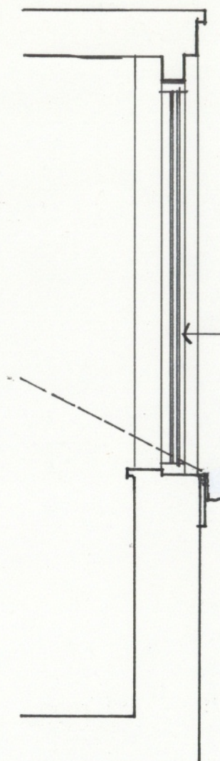
SECTION A-A. SCALE: 1:20 @ A3.
