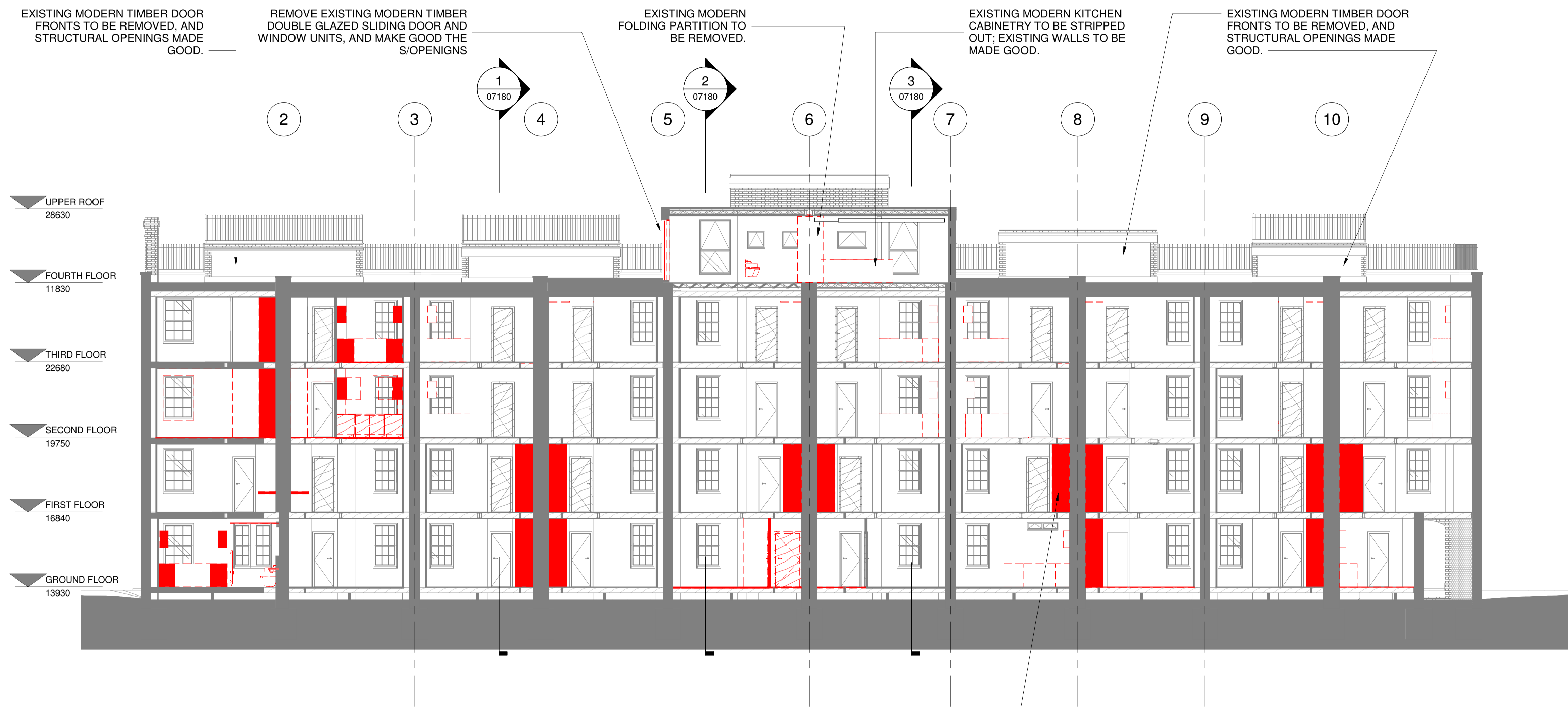
1 DEMOLITION - SECTION E 07181 05120 1:100
