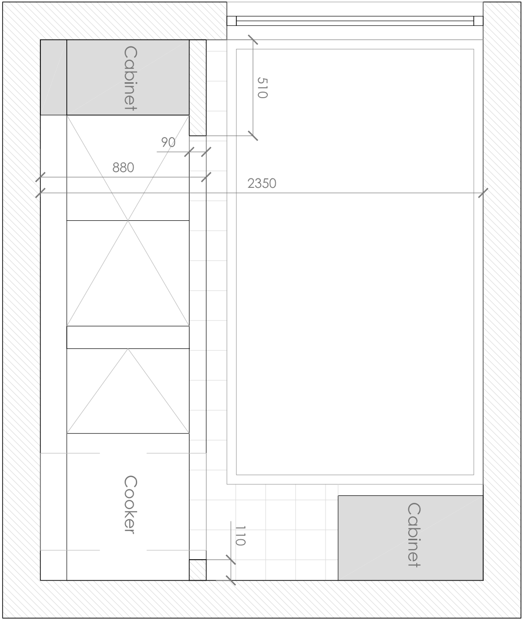
ELEVATION A
