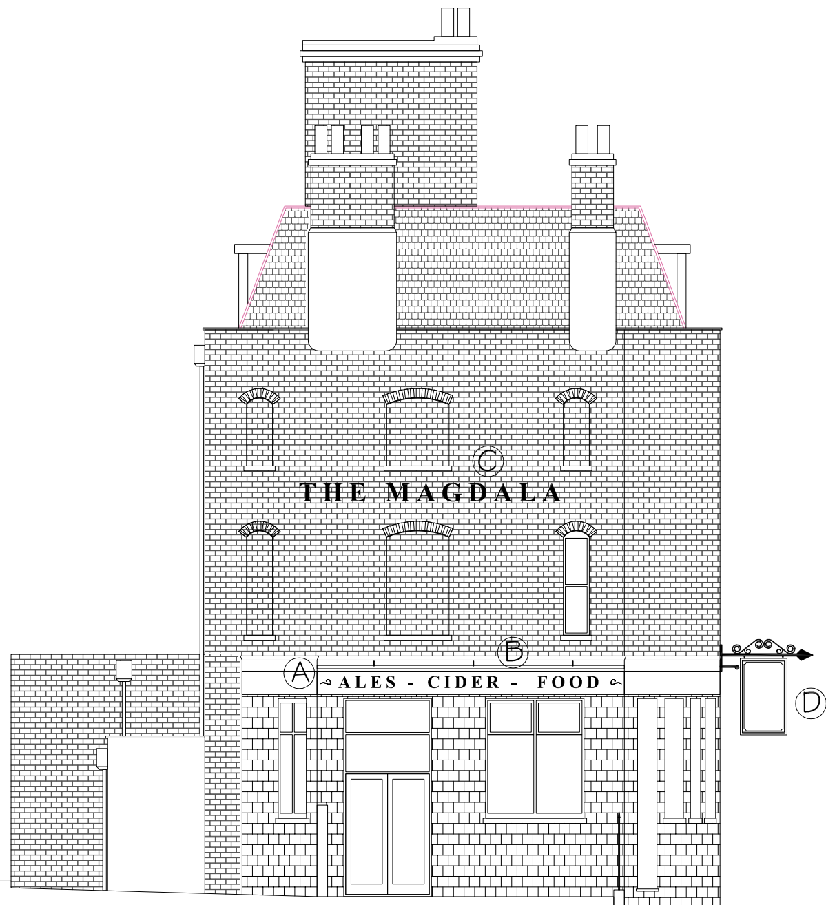
END ELEVATION : Scale: 1:100 @ A3
