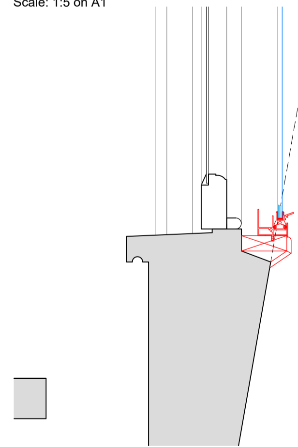
Section G-G Scale: 1:5 on A1
