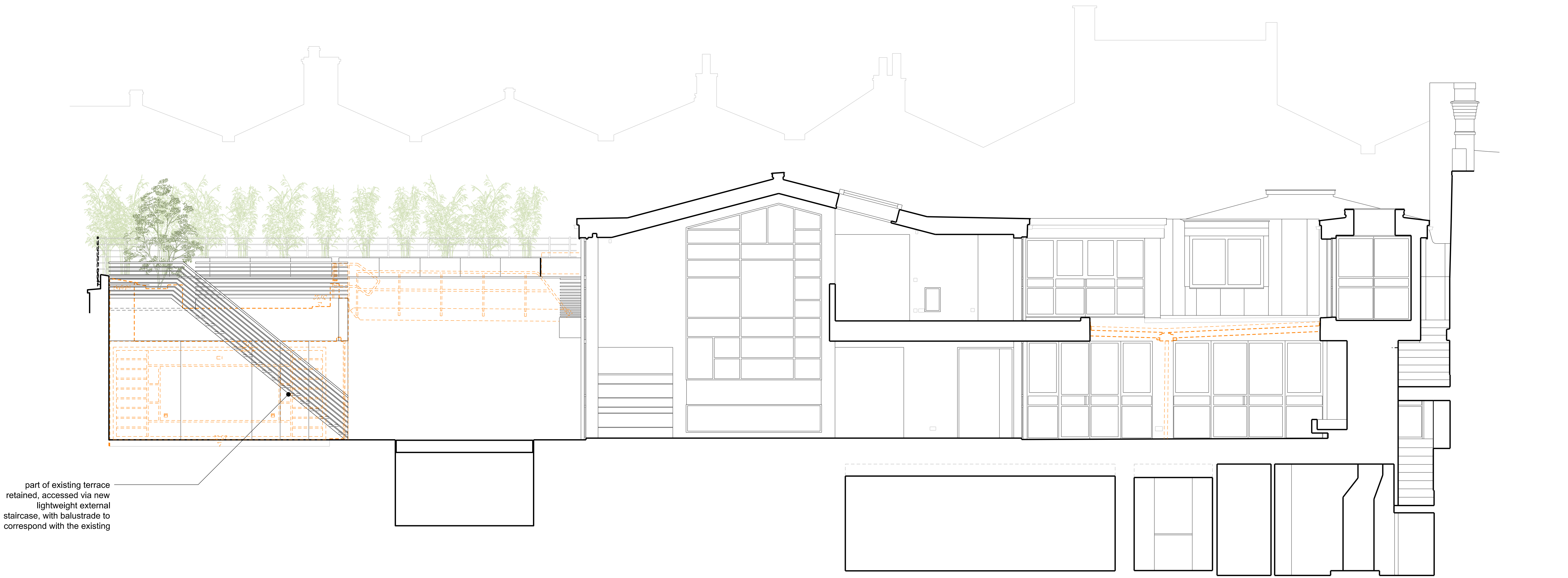
01 Section BB Scale 1:50 @ A1 / 1:100 @ A3
