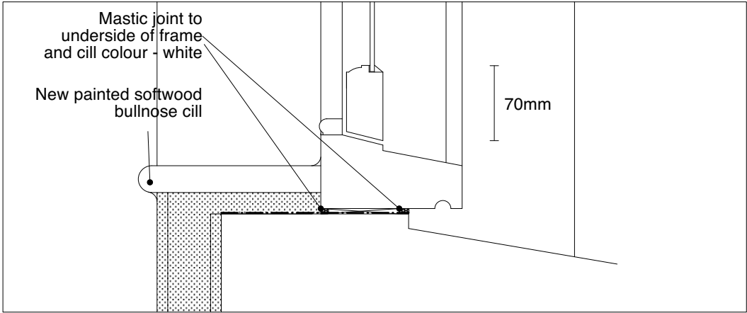
Cill
