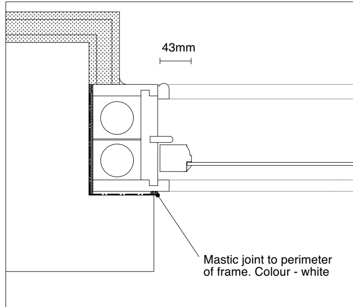
Jamb
