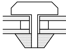
Existing Door - Jamb 1:2 @ A3
