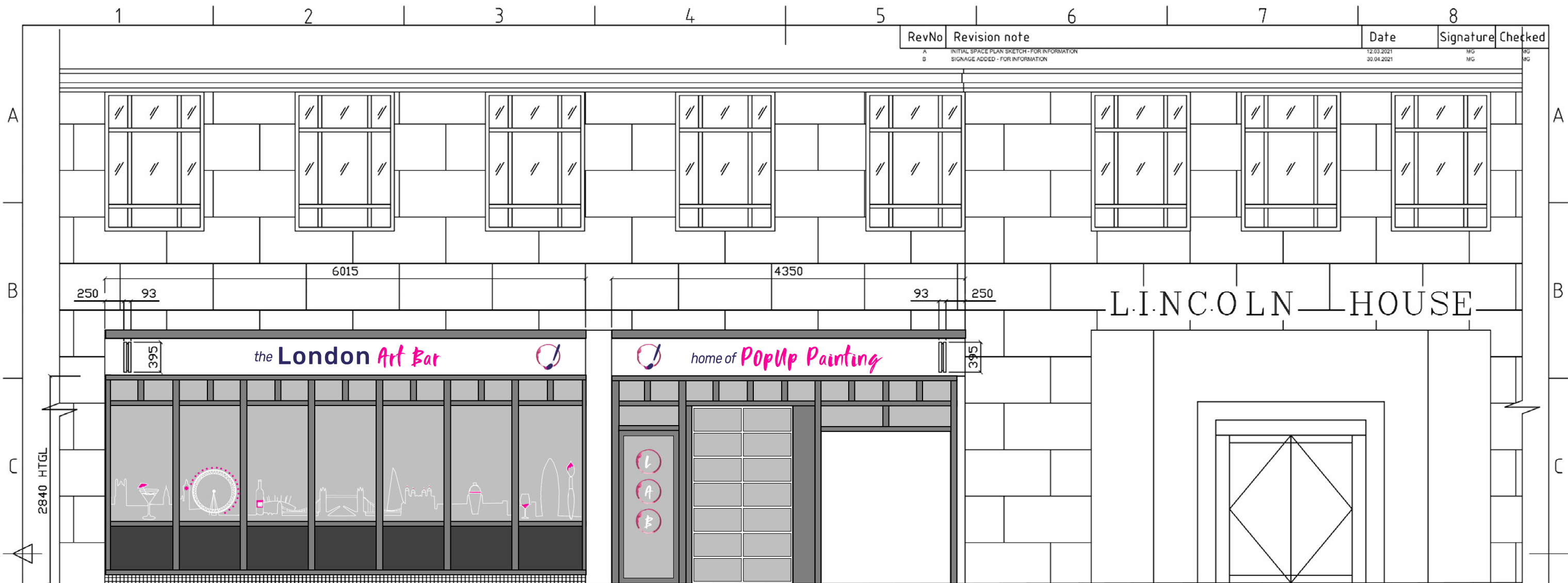
A EXTERIOR ELEVATION - SCALE: 1:50@A3
