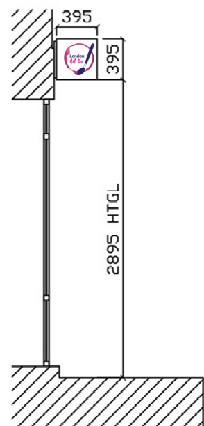
B EXTERIOR SECTION - SCALE: 1:50@A3
